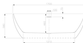
SEZIONE F-F
