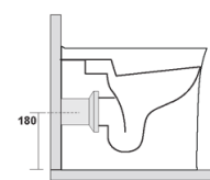
tubo di raccordo a parete art. 7539
