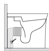
max. 140 / min. 60 con curva art. 900104
