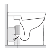
max. 230 / min. 170 con curva art. 7619
