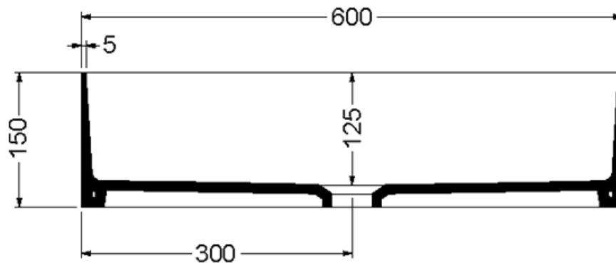
SEZIONE
