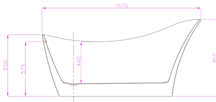
SEZIONE F-F
