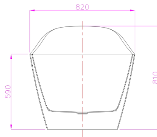
SEZIONE G-G
