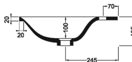
SEZIONE A-A SECTION A-A
