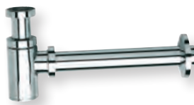
Siphon de lavabo/bidet laiton design droit luxe 35 cm, 1"1/4, spécialement adapté pour faibles encombrements CHROME | MS 3651 | 128€
