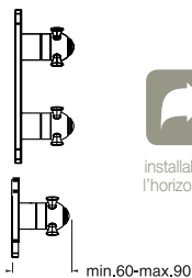
Façade laiton 2 sorties façade laiton pour bati PD 70200 CHROMÉ | XC 88251 | 849€
