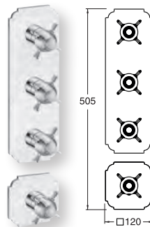
BATI 3 sorties rail, boîtier thermostatique, 3 robinets d'arrêt PD 70300 | 799€
